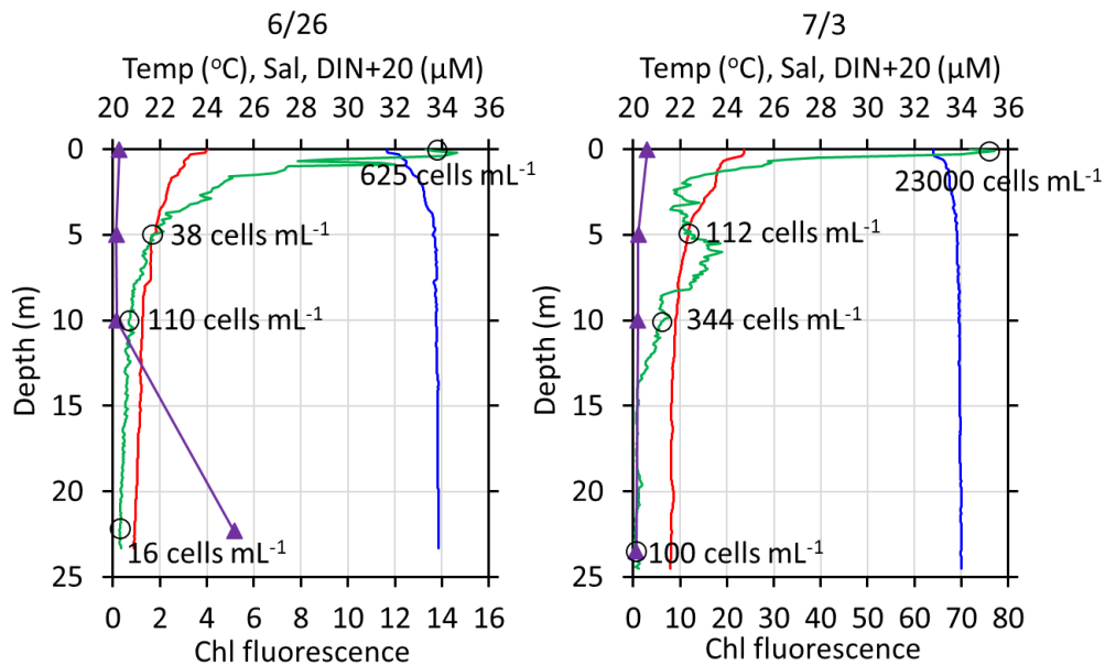
図 4. 2018 年 6 月 26 日および 7 月 3 日の Stm. U6 における水温 (赤線), 塩分 (青線), クロロフィル蛍光強度 (緑線), DIN 濃度 (紫線), K. mikimotoi 細胞密度 (白丸) の鉛直分布。
