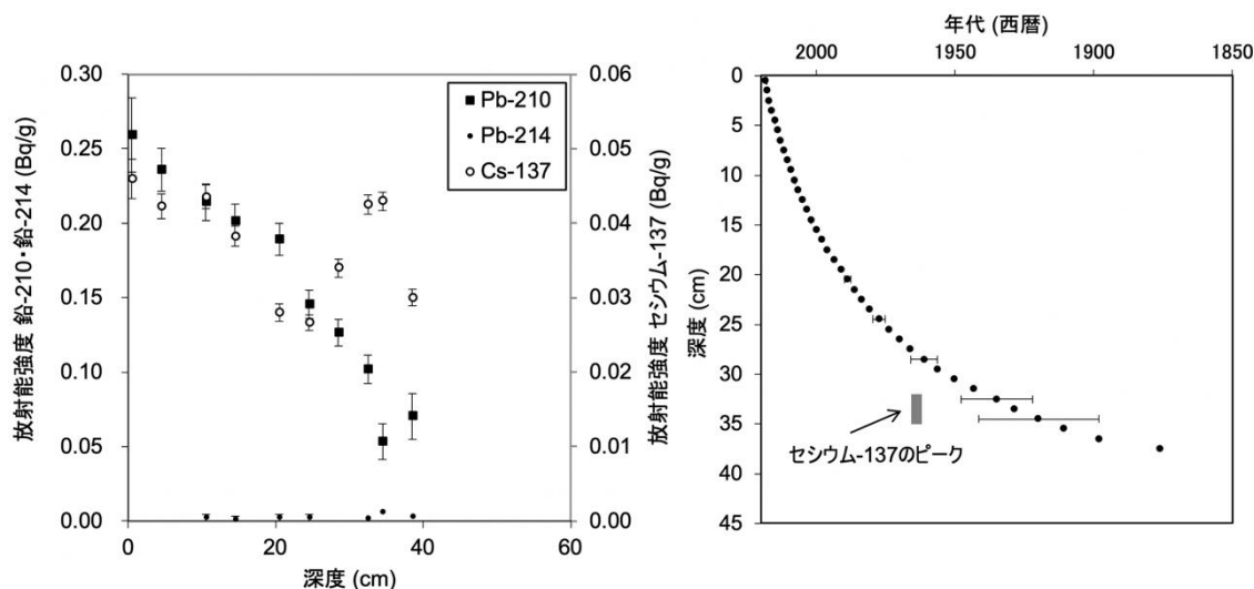
図2 鉛-210、鉛-214とセシウム-137の放射能強度（左）とCRS (Constant Rate of Supply)モデルによる年代-深度分布（右）
