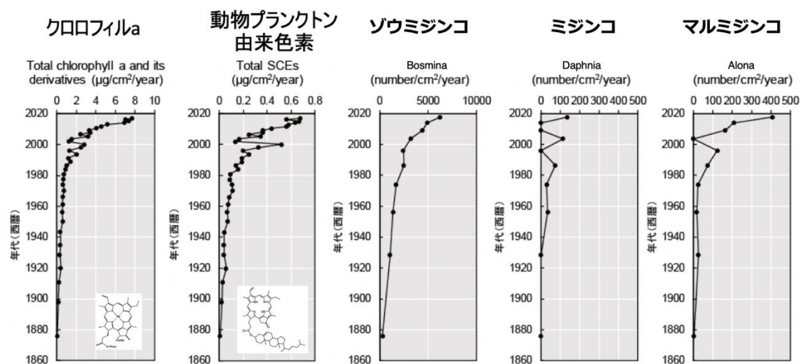
図 2 山中湖における過去 150 年間の色素及び動物プランクトン（ミジンコ類）の年間堆積量の変化
