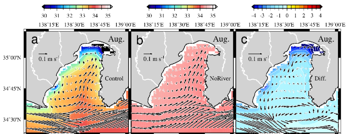
図 2 駿河湾における 8 月の海面の塩分と流れの月平均気候値. (a)Control 実験, (b)NoRiver 実験, (c)Control 実験と NoRiver 実験の差分.
