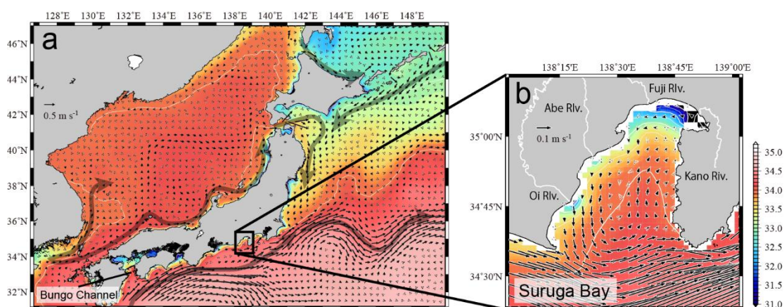
図 1 (a)日本周辺高解像度モデルの計算領域と(b)駿河湾における 2008 年 1 月 1 日から 2014 年 12 月 31 日までの海面における塩分と流れの平均場 (Control 実験). 図 1a の太い黒矢印は海況シミュレーションによって表現された日本周辺海域の主な海流（黒潮, 黒潮続流, 東韓暖流, 対馬暖流, 津軽暖流, 宗谷暖流, 親潮）を模式的に示している。図 1b の陸上の白線は一級系の河川を示しており, “Kano Riv.”, “Fuji Riv.”, “Abe Riv.”, “Oi Riv.”はそれぞれ, 狩野川, 富士川, 安部川, 大井川である。
